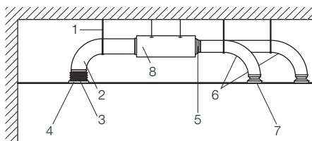
Типовая схема подключения круглых вентиляционных каналов
